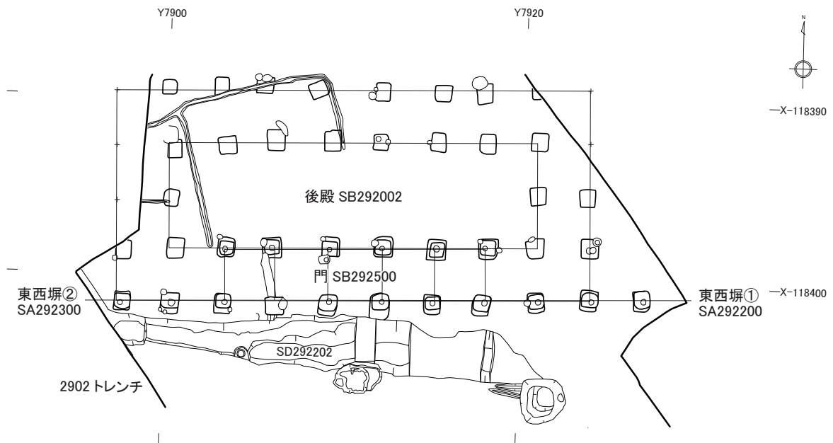
図5 後殿 SB292002 と門 SB292500 の重複
