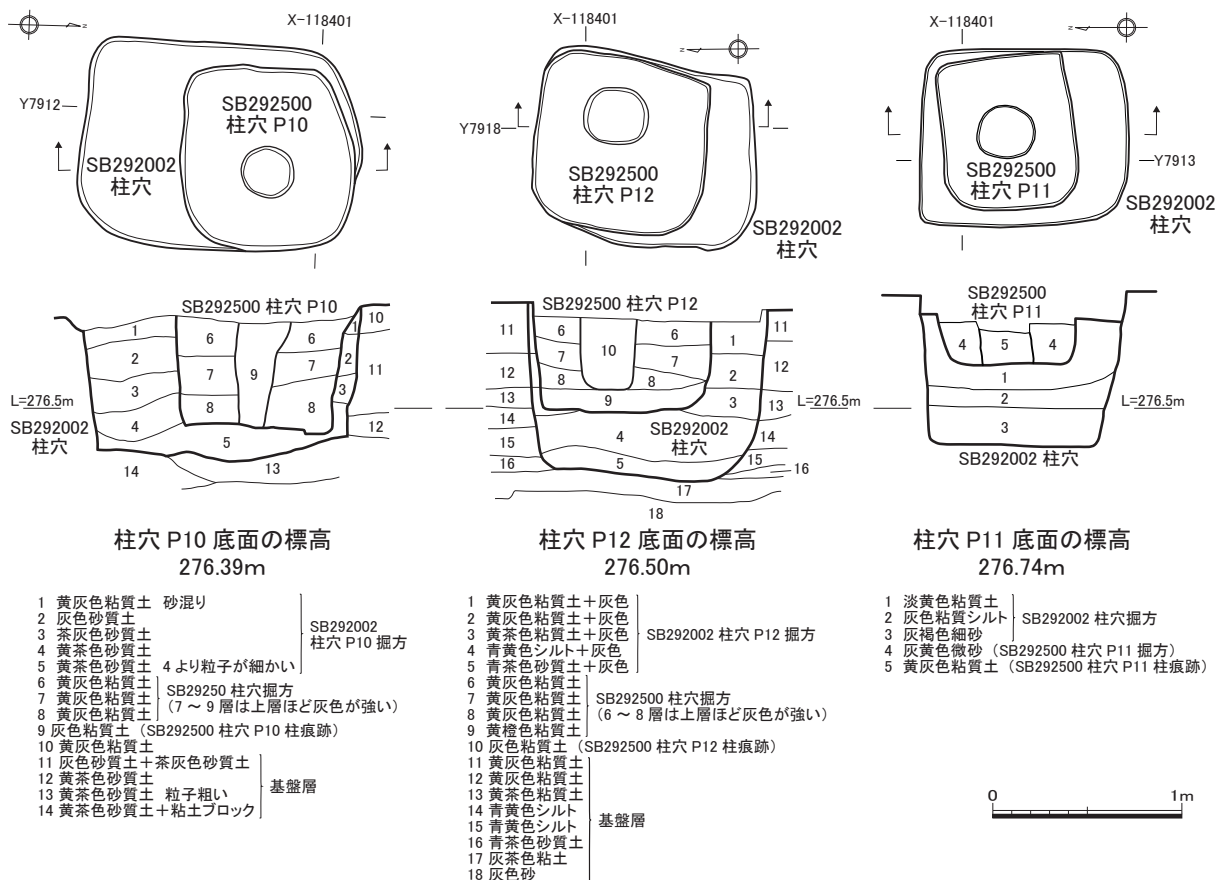
図3 後殿 SB292002・門 SB292500 柱穴平面図・断面図
