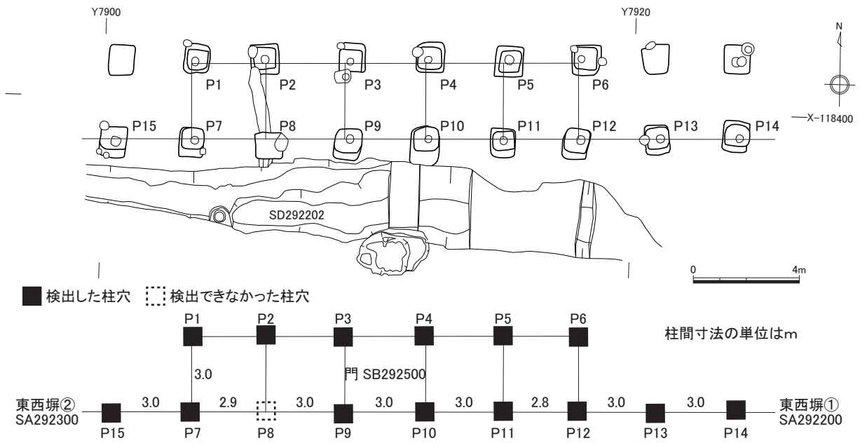
図4 門 SB292500 平面図
