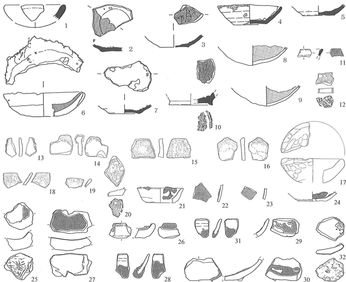
第1図 鉄生産関連遺物 1
