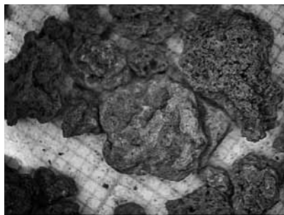
図4 低温酸化した柏原遺跡大淵スコリア 縄状によじれた厚皮膜、直面状破断面、多角形状～楕円形気孔、気孔間壁が頑丈なのが特徴。このスコリアの場合、内部には面積率が 50% 以下の気孔群がある。その形態は球形～多角形が多く、気孔間壁が厚くて頑丈である。方眼の 1 目盛は 1 mm。
