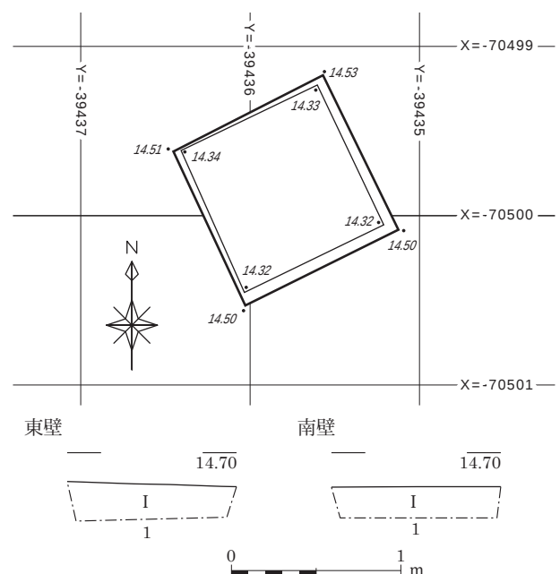
第 28 図 第 14 次調査 TP-1 平断面図 (1/40)
