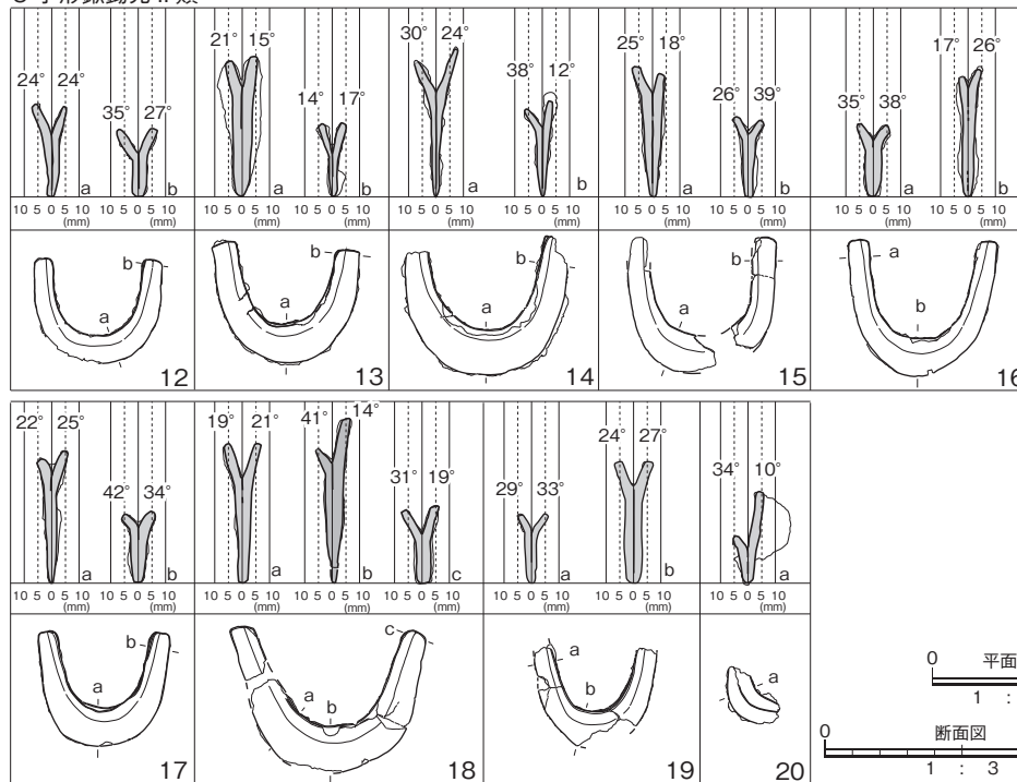
図11 V字溝の断面形状1
