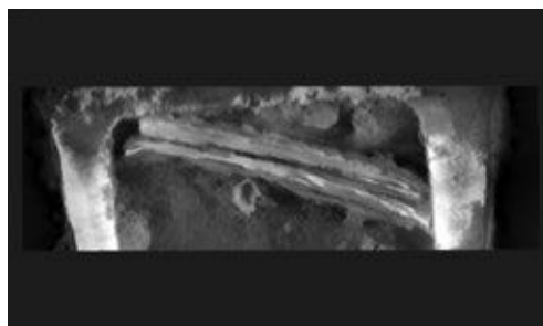
第124図 鑄造鉄斧袋部内部のCT画像
