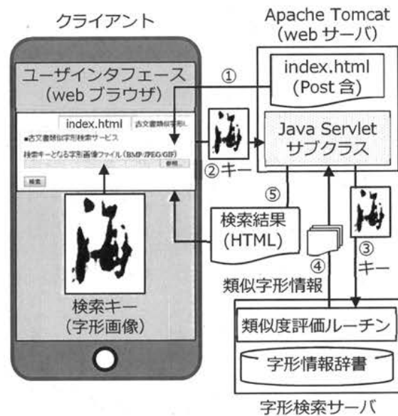
図 9 字形検索 web アプリケーションの設計 Figure 9 Design of web application for character pattern retrieval.
