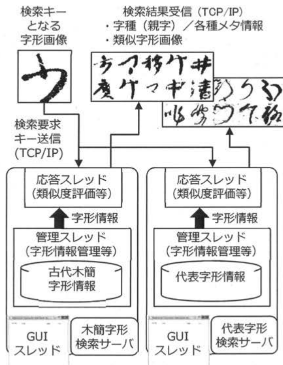
図 8 クライアント・サーバ方式のプラットフォームを用いた字形横断検索
