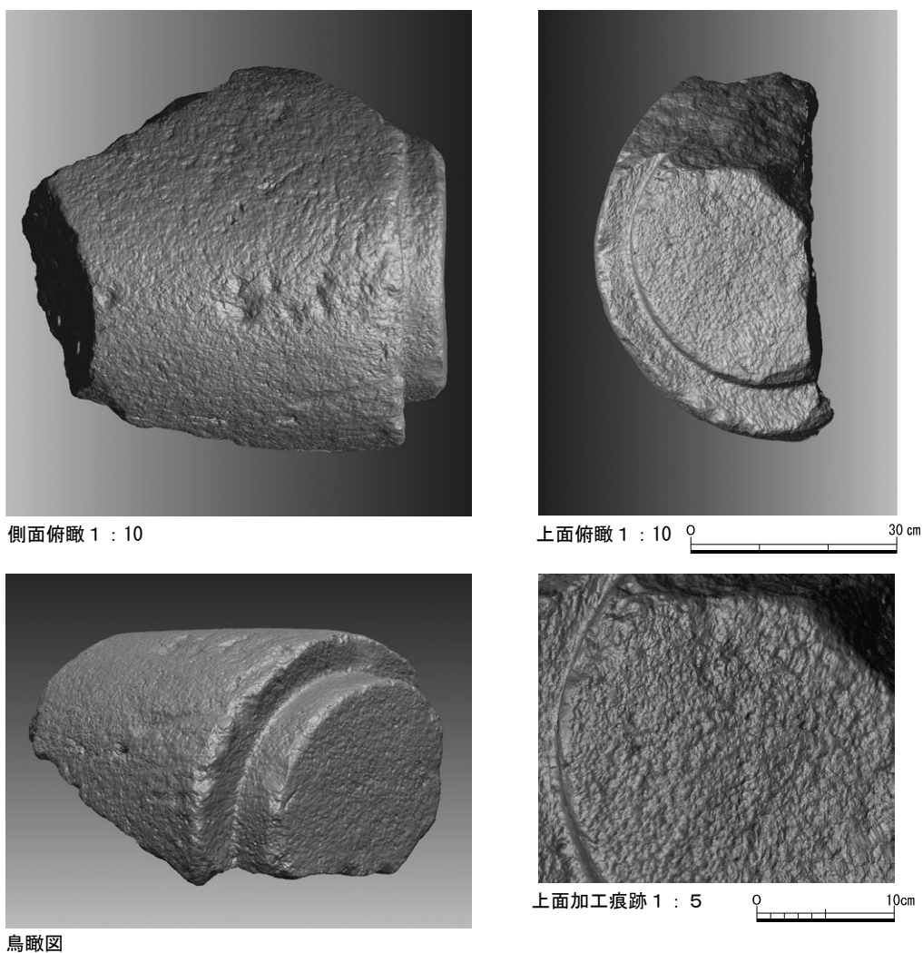
図8 飛鳥寺出土亀山石製不明石造物三次元レーザー計測画像
