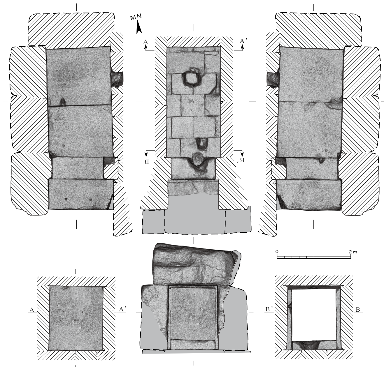
図1 平野塚穴山古墳石槨三次元レーザー測量図 1 : 60
