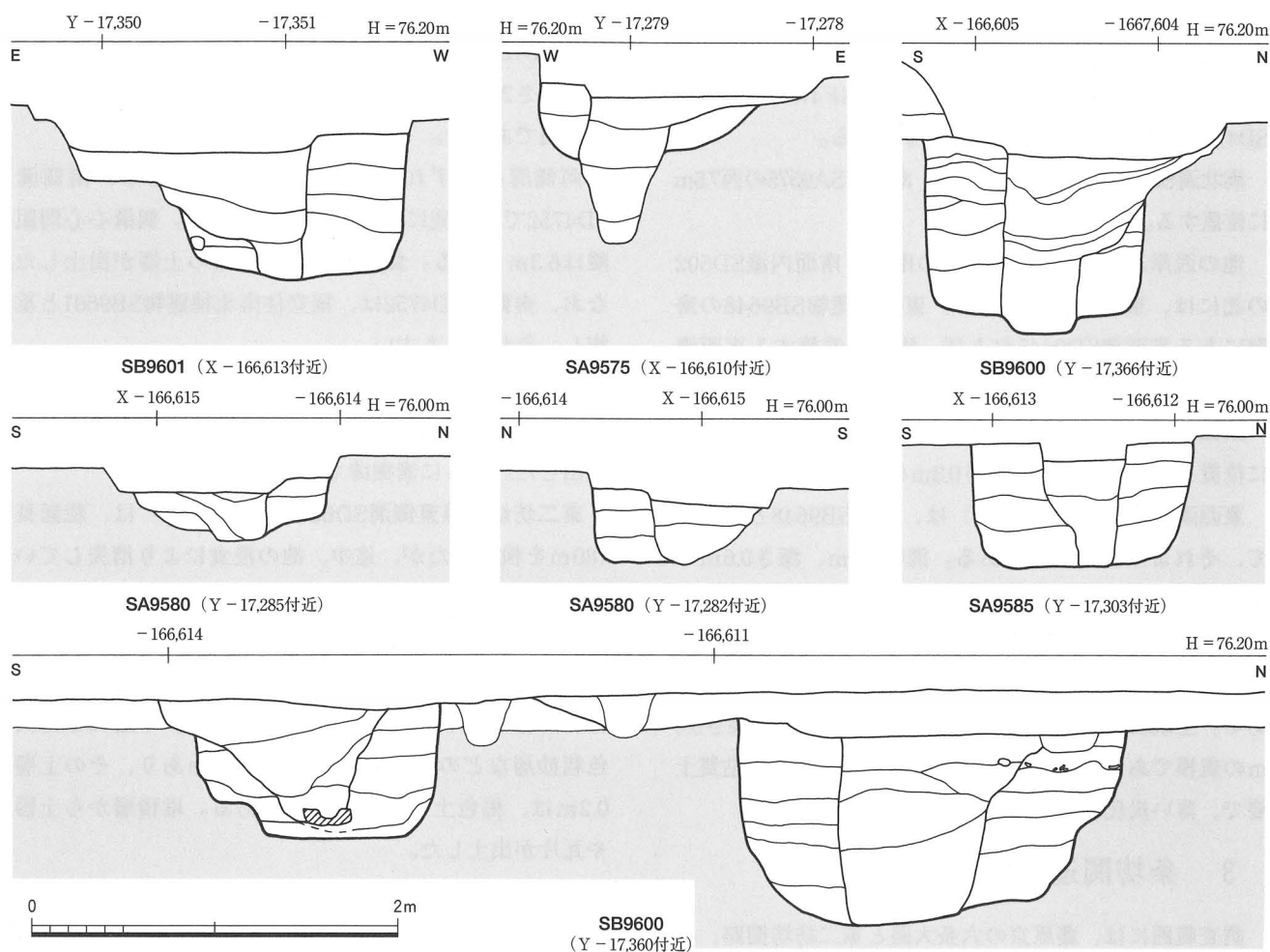
Fig. 6 建物・堀の柱穴断面図 1:40
