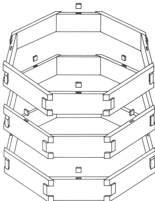
図11 井戸枠組み上げ模式図
