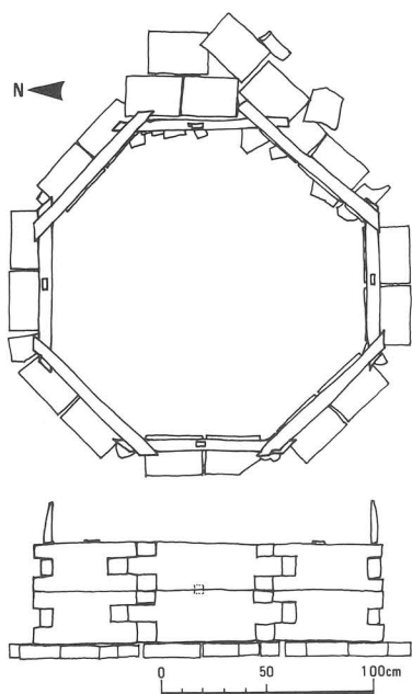
図10 井戸枠実測図 〈多角形井戸の出土例〉
