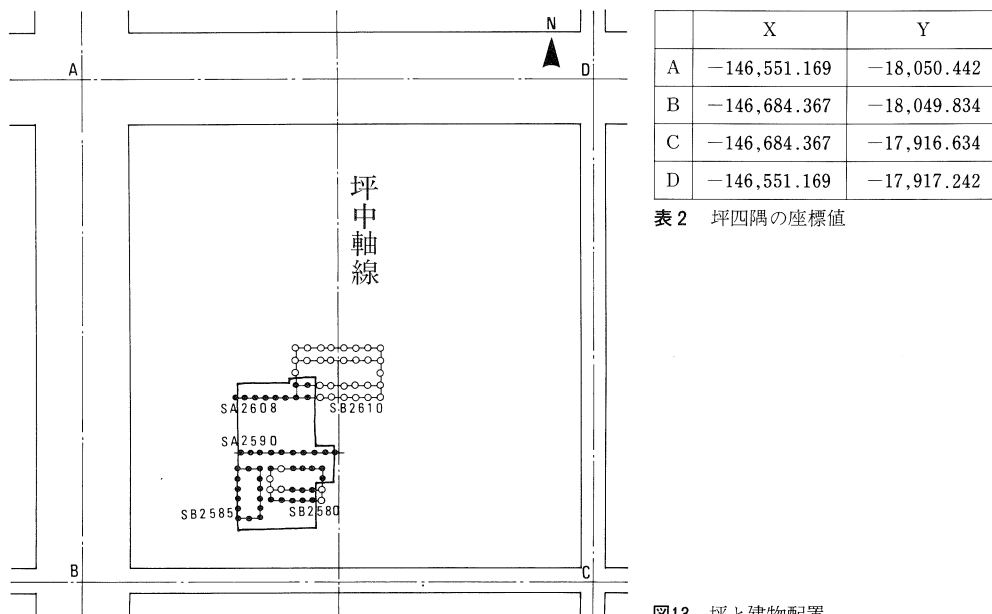
図13 坪と建物配置
