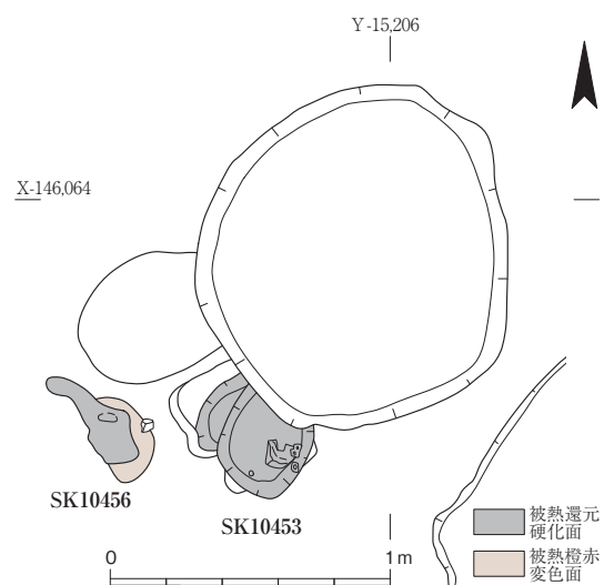
第16図 鉄鍛冶遺構SK10453・10456 平面図 1:30
