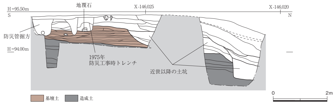
第24図 Ⅲ区西壁土層図 1:80
