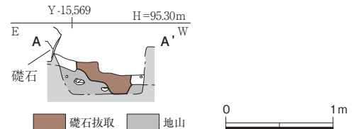
第26図 Ⅲ区礎石断割土層図 1:50
