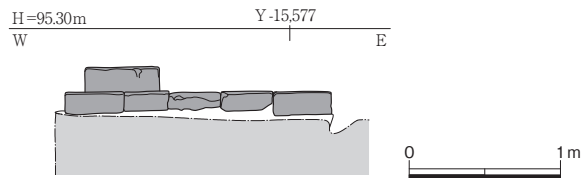
第25図 Ⅲ区基壇外装立面図 1:50
