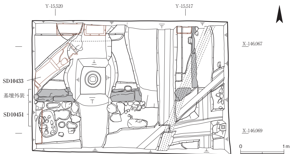
第8図 基壇東南隅 (東拡張区) 平面図 1:50
