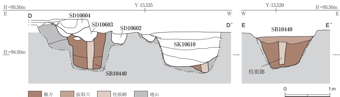
第12図 SB10440柱穴断割土層図（左：D-D'、右：E-E'） 1：50
