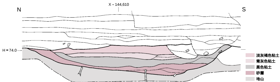
图10 SD985 断面图 (Y = -20,102) 1:40
