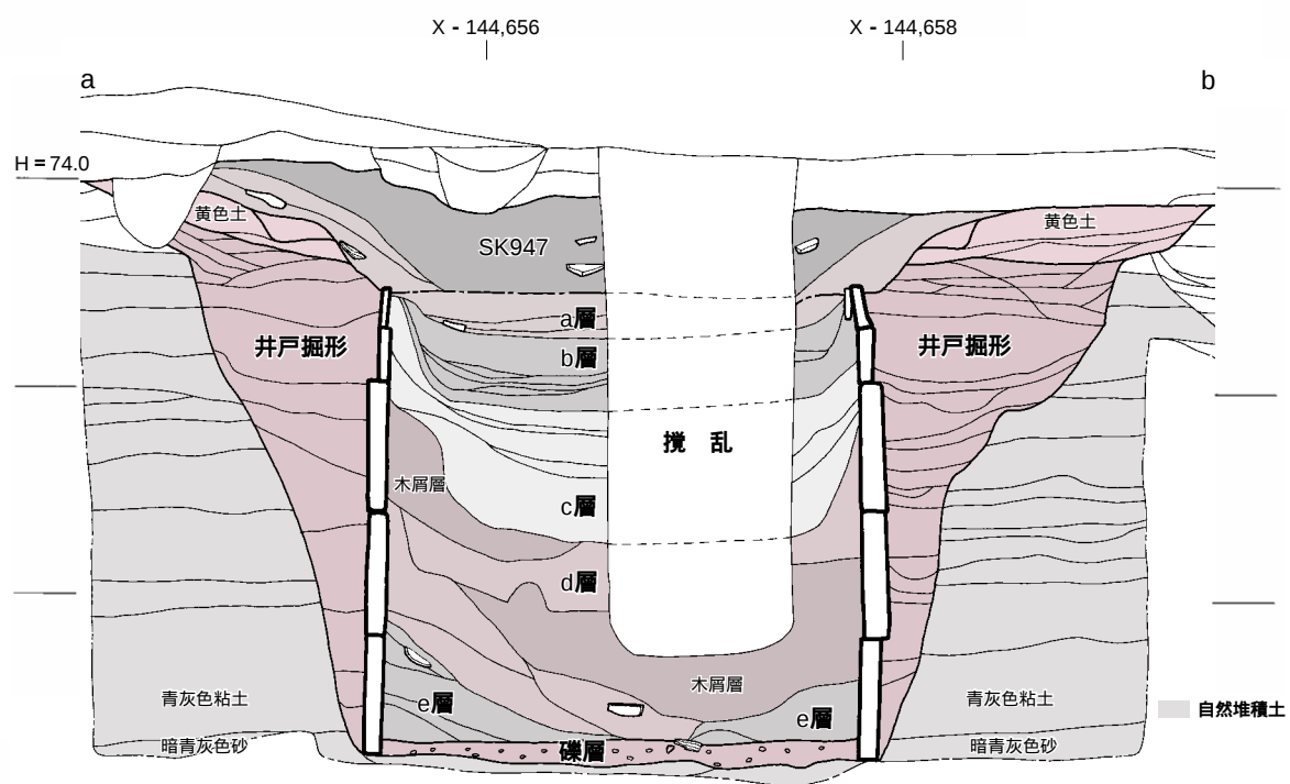
图15 SE950 断面図 1:40
