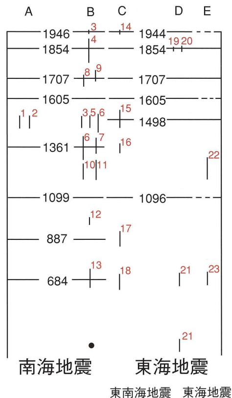
Fig.52 南海地震と東海地震の発生年表
