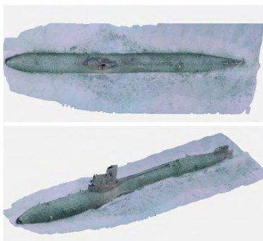
図3-6-5 静岡県下田市沖に沈む特殊潜航艇「海龍」三次元画像 海龍や潜航艇の形状が把握でき、三次元画像から平面図等を作成することも可能である(上)。さらに、海龍や潜航艇の形状をイメージしやすい画像(下)を作成することも可能であることから、多くの活用における利用も期待される。
