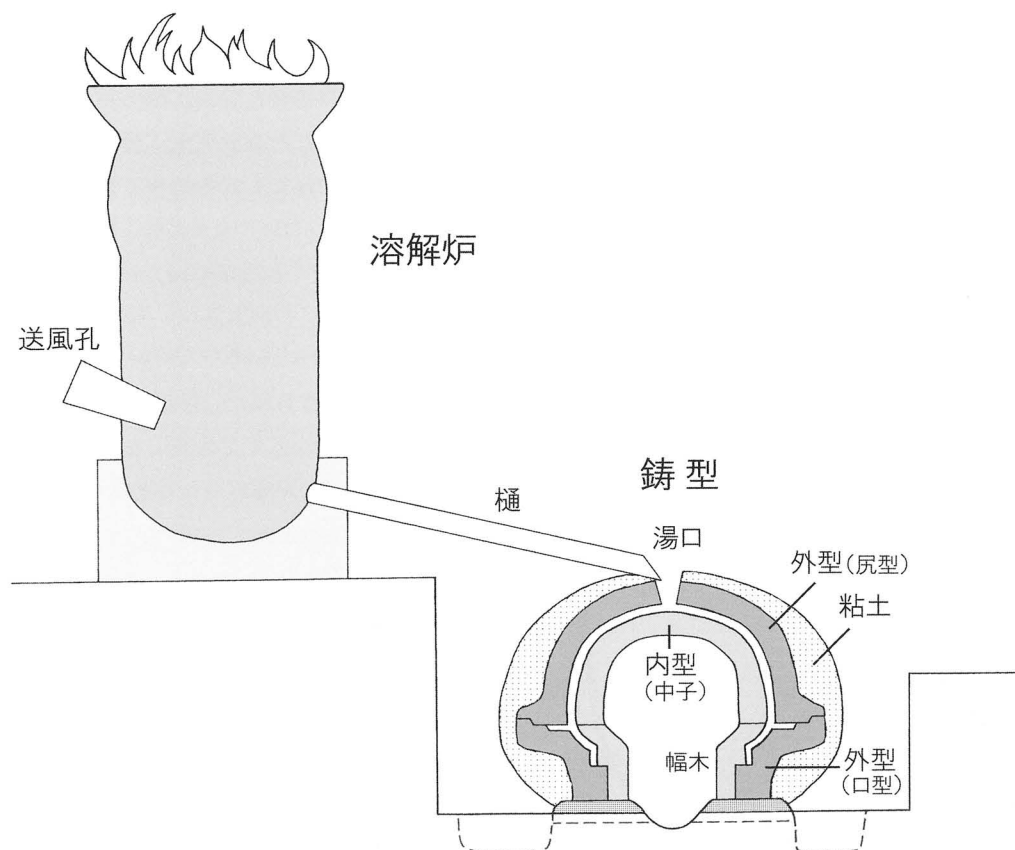
Fig.26 鉄釜鑄造作業復原模式図
