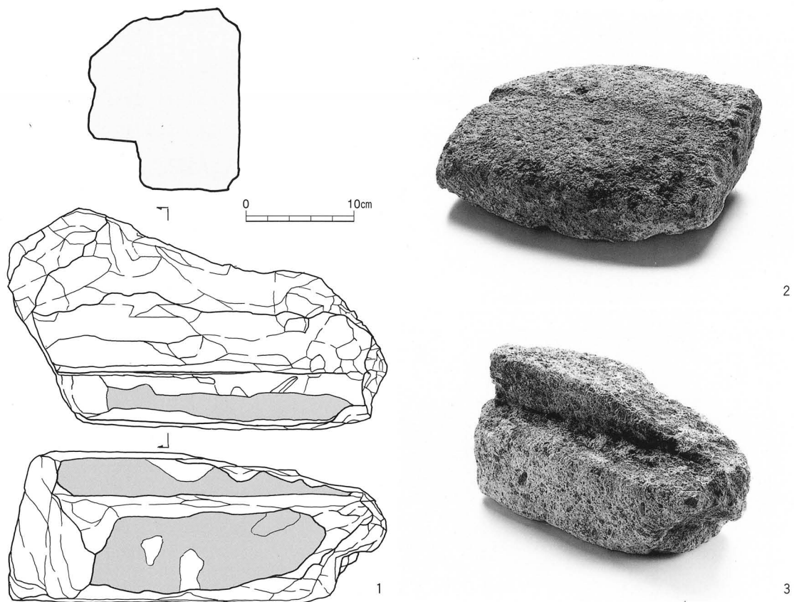
第18図 石材
