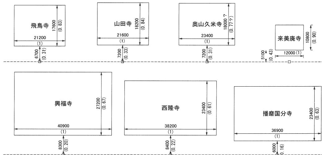
fig.24 灯籠・金堂位置関係模式図(単位:mm) 1:1000
