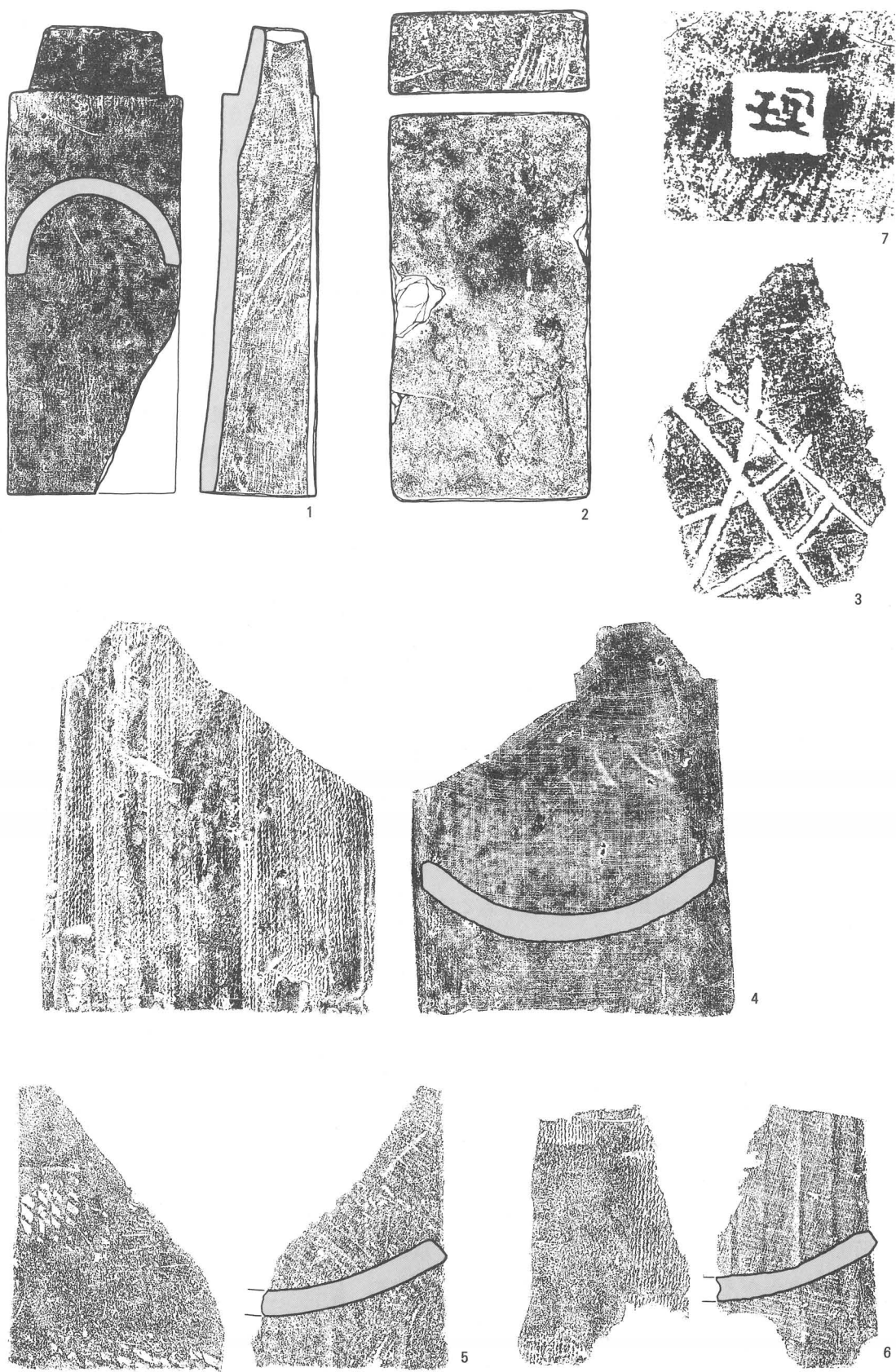
Fig. 7 瓦罍実測図・拓影 1・2・4～6-1:5 3-1:2 7-3:4
