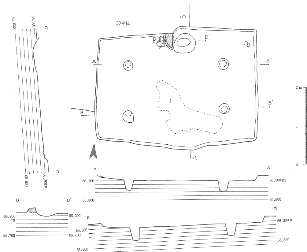
第78図 29号住居跡実測図
