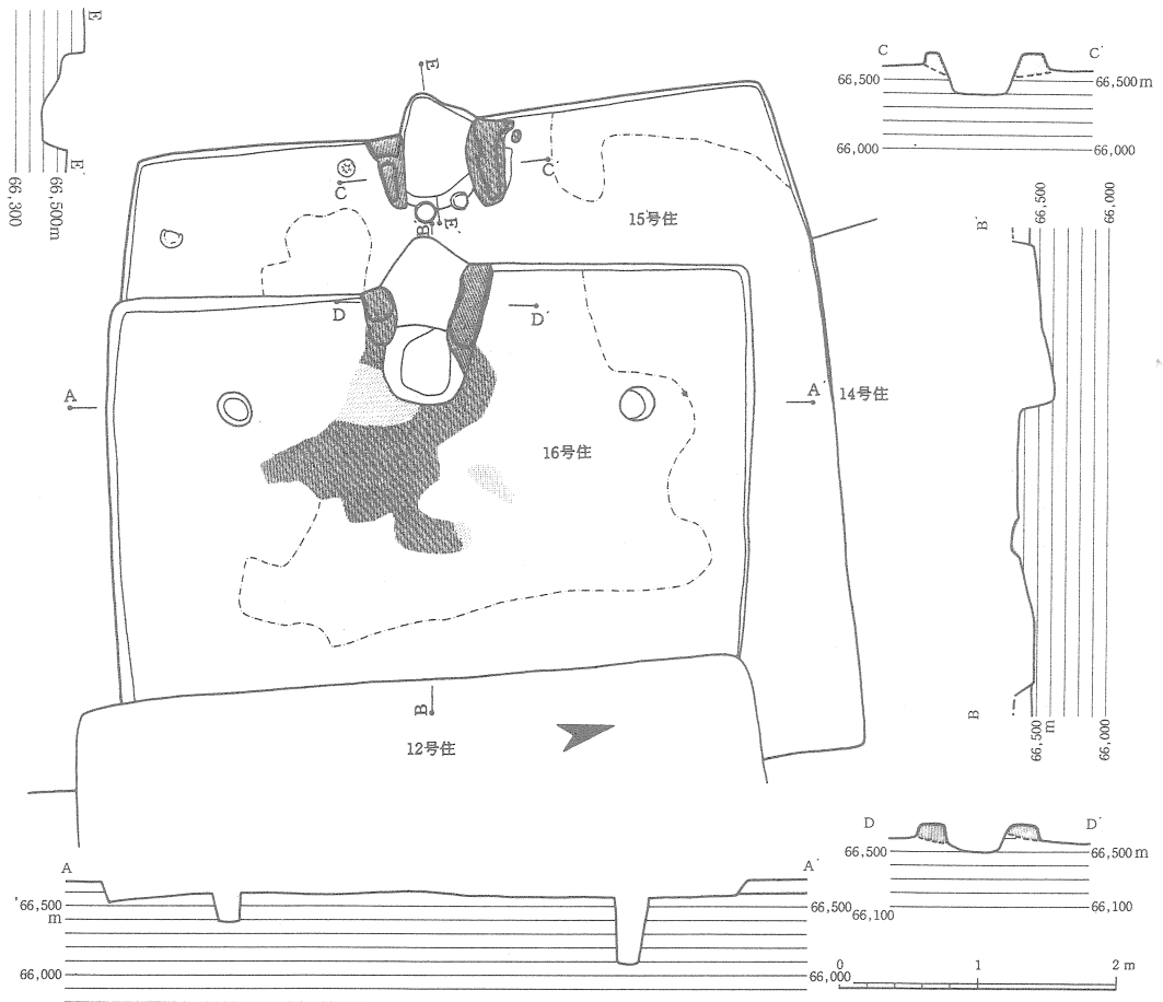
第61図 15号・16号住居跡実測図
