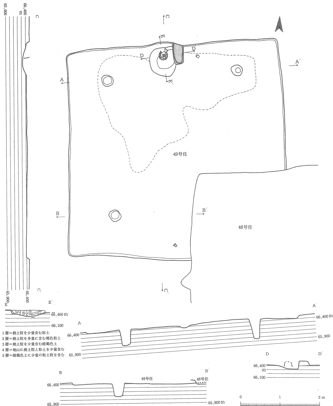
第100図 49号住居跡実測図
