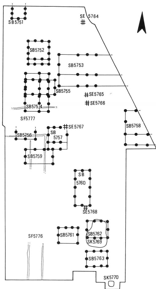
fig.7 遺構配置図
