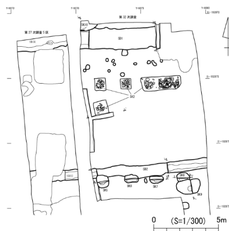
第8図 北辺溝平面図 (文献7から作成)
