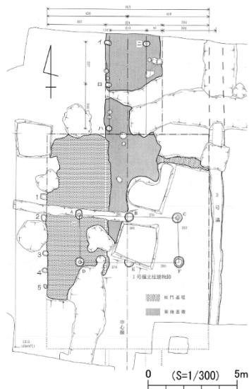
第7図 東門平面図 (文献2に加筆・修正)
