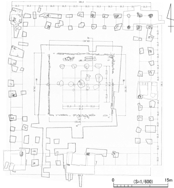
第5図 塔平面図 (文献1に加筆・修正)
