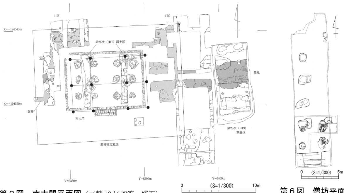
第3図 南大門平面図 (文献10に加筆・修正)
