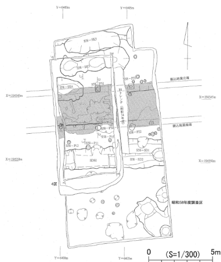
第4図 南辺築地・大溝平面図 (文献10に加筆・修正)
