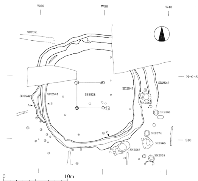
第8図 Ⅲ期 SB2528 (SD2541・2542) 建物 (大和町 2003)
