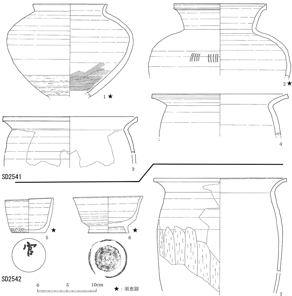
第9図 SB2528 (SD2541・2542) 出土遺物 (大和町 2003 に加筆)
