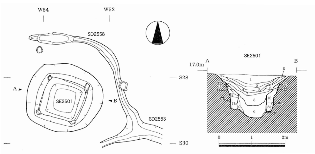
第7図 II B期 SE2501 井戸 (大和町 2003)
