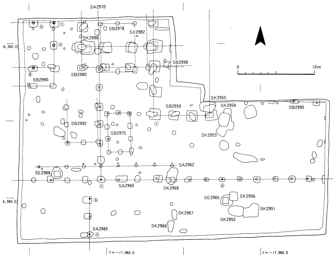
fig. 8 遺構配置図
