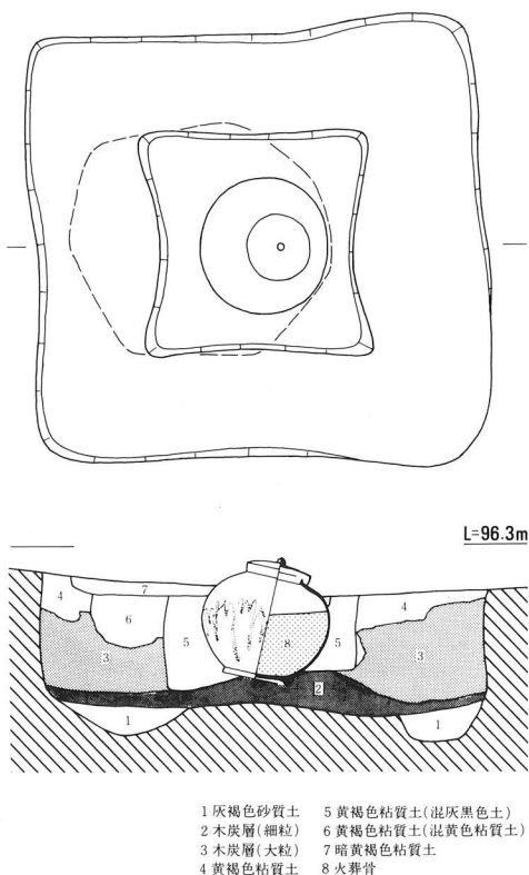
fig. 13 SX1075遺構図
