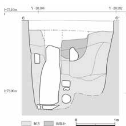
図7 掘立柱 SX1150 断面図
