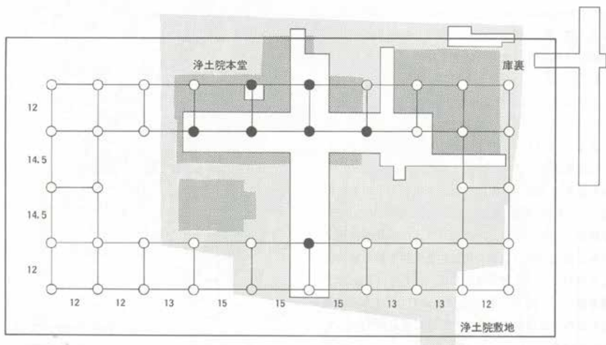
図8 薬師金堂復元図
