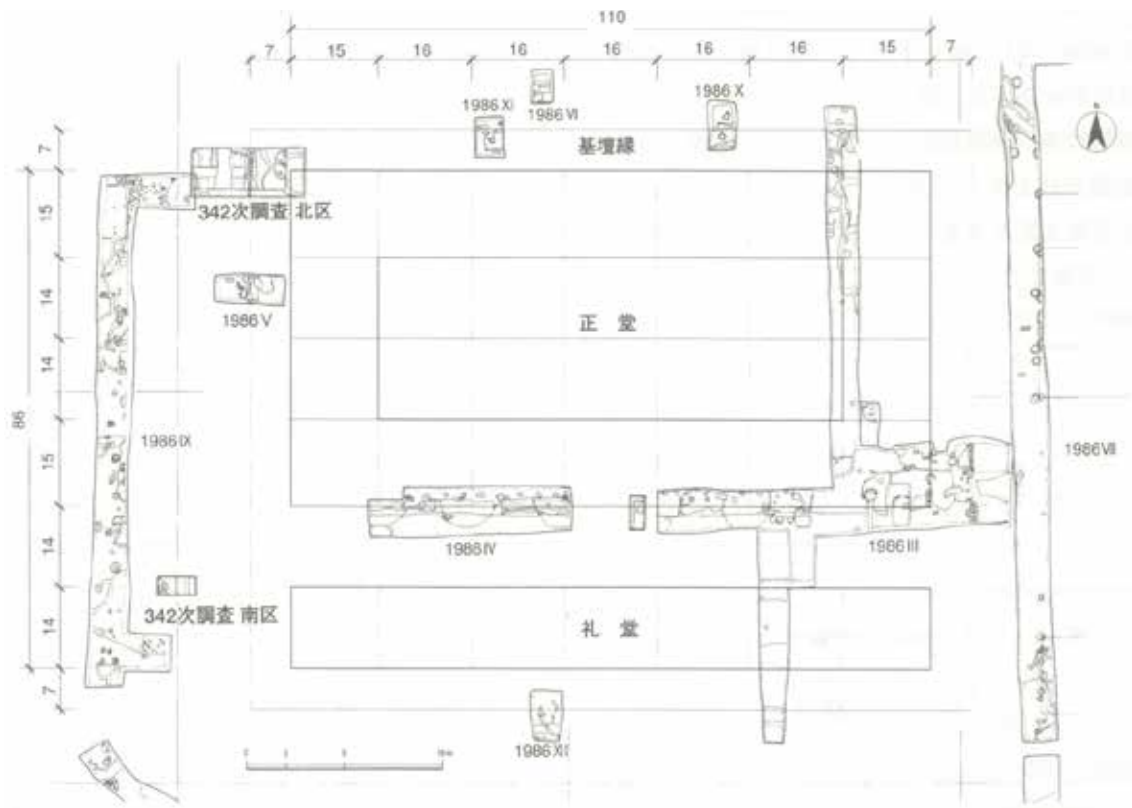
図3 四王堂の復元図
