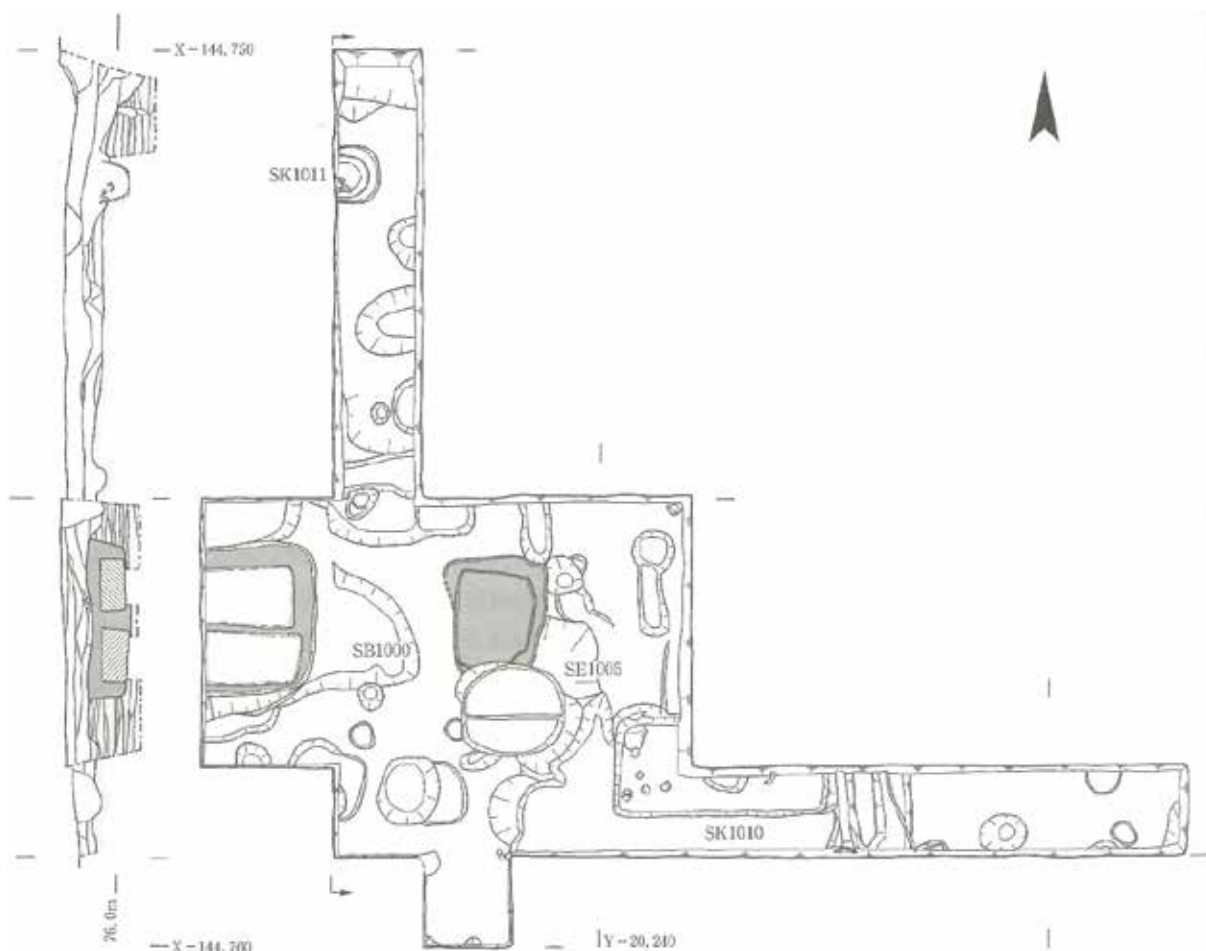
図5 第409次調査区平面図・断面図
