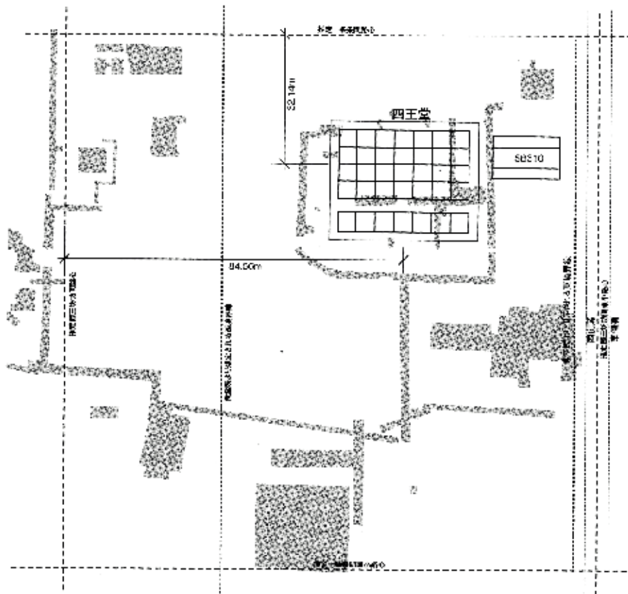
図4 四王堂配置復元図
