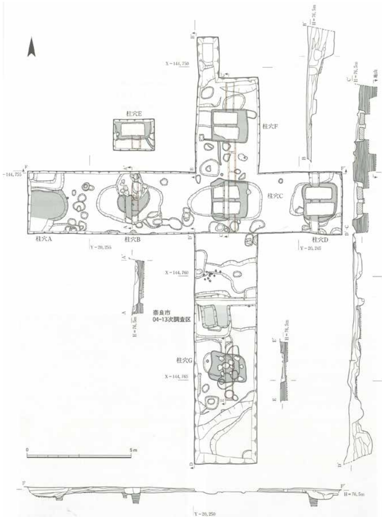
図7 第422次調査区平面図・断面図
