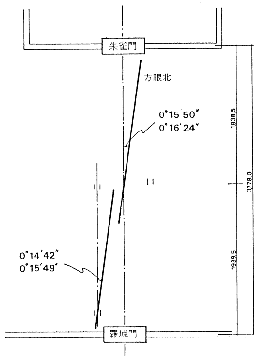
fig.26 朱雀大路中軸線方位概念図
