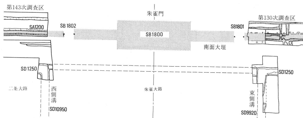
fig.27 平城宮第130・143次調査遺構図
