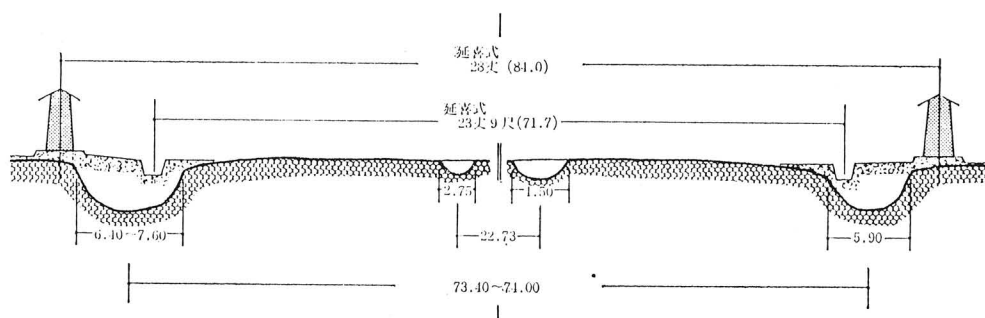
fig.23 朱雀大路横断面模式図
