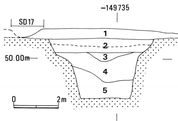
fig.27 SE 18土層図 1 : 50
