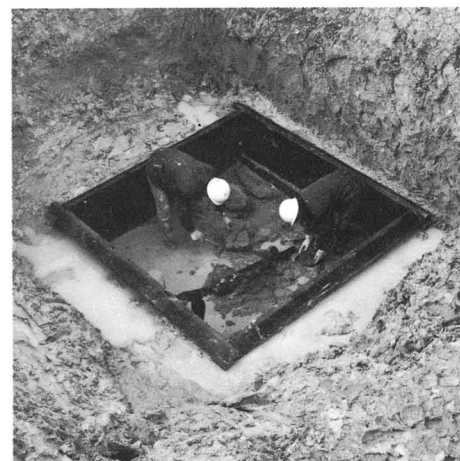
fig. 27 校倉の校木を使った井戸枠 平城宮跡第一次大極殿地区検出
