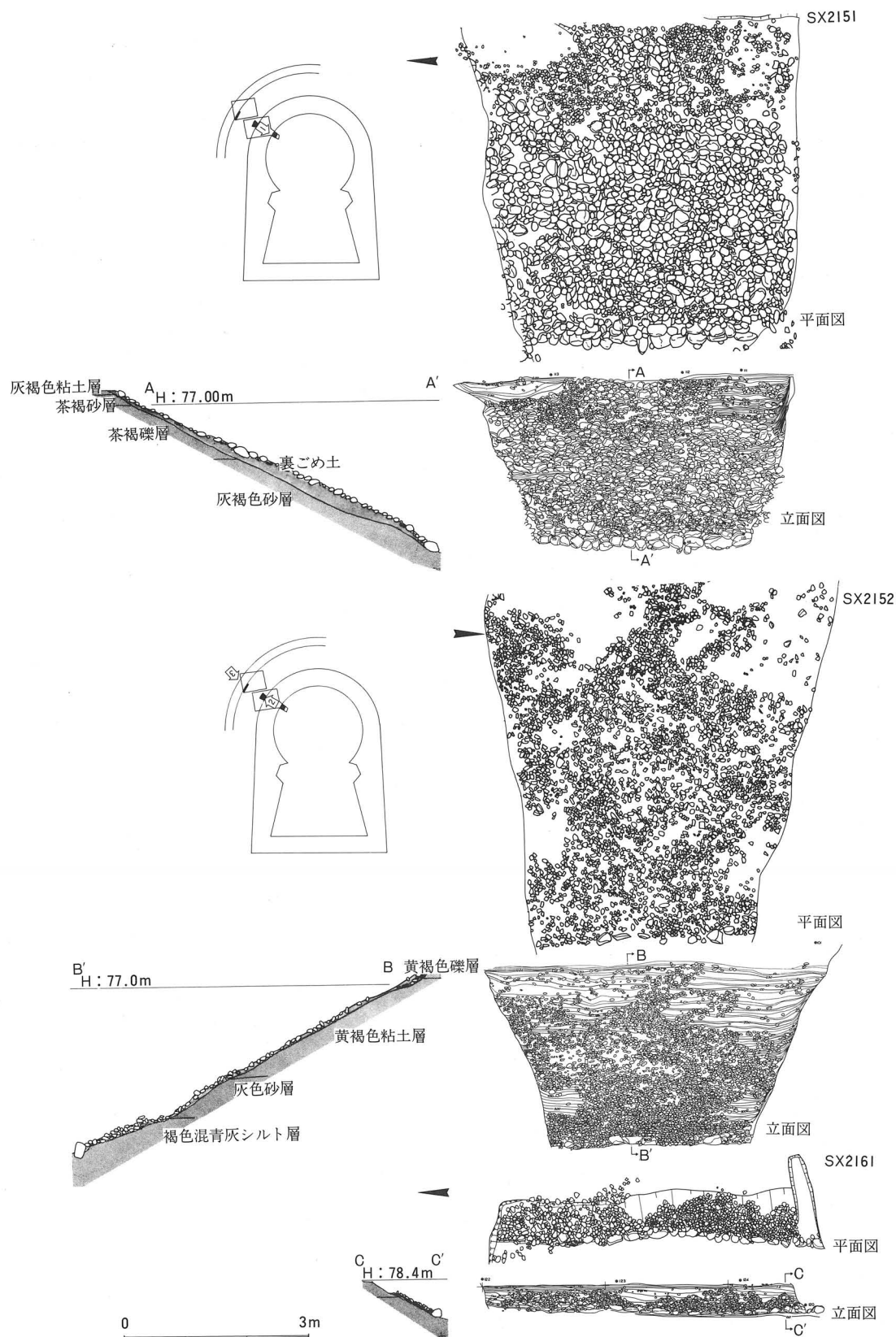
fig. 9 葦石実測図
