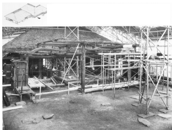
重要文化財・旧太田家住宅主屋の復旧工事
