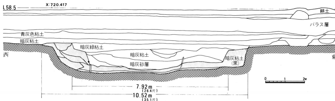
堀河断面模式図（北側トレンチ）
