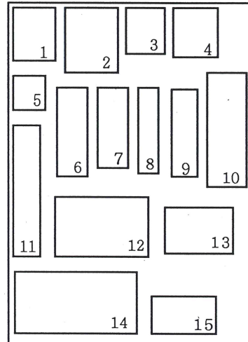
第2図 今金ー北桧山地 域産出の有孔虫 化石 (その1: 35ページ)
