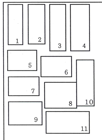
第4図 今金ー北桧山地 域産出の有孔虫 化石 (その3: 37ページ)
