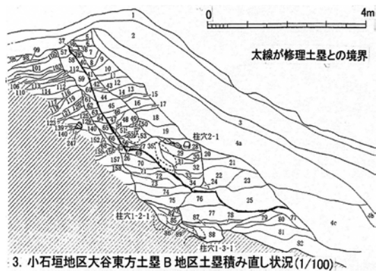
図31 小石垣地区大谷東方土塁積み直し状況（入佐・小澤2010）
