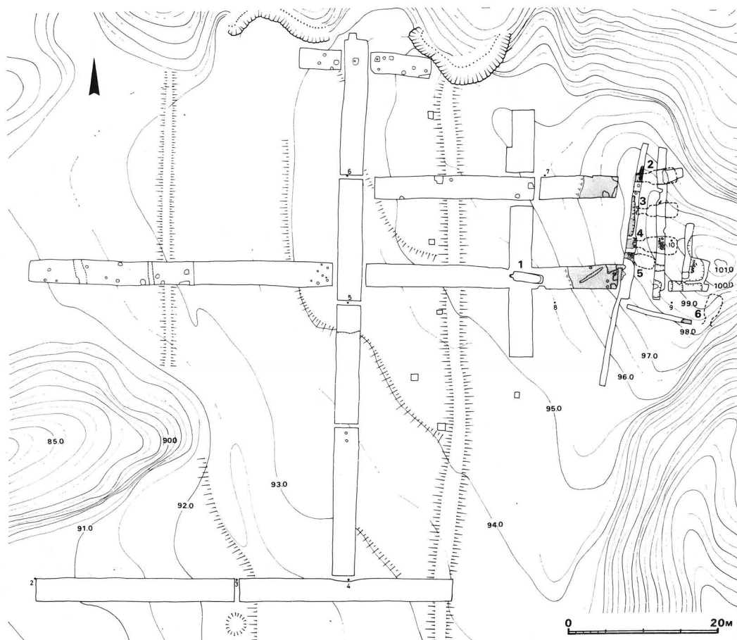
第3図 第2号地点—押熊瓦窯—遺構配置図
