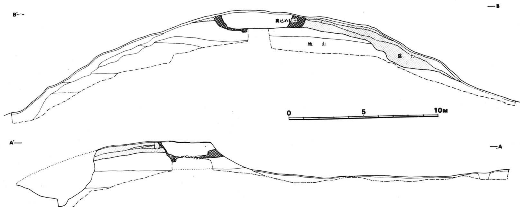
第13図 音乗谷古墳 墳丘断面図
