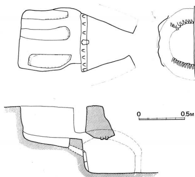
第9図 音如ケ谷瓦窯遺構図
