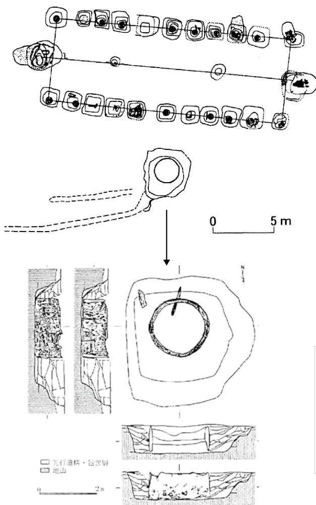
図2 池上曽根遺跡の大型建物と大型井戸
