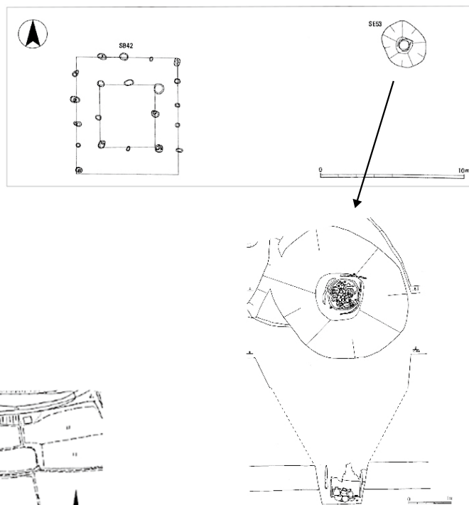
図4 三重県古響通りB遺跡の儀礼空間
