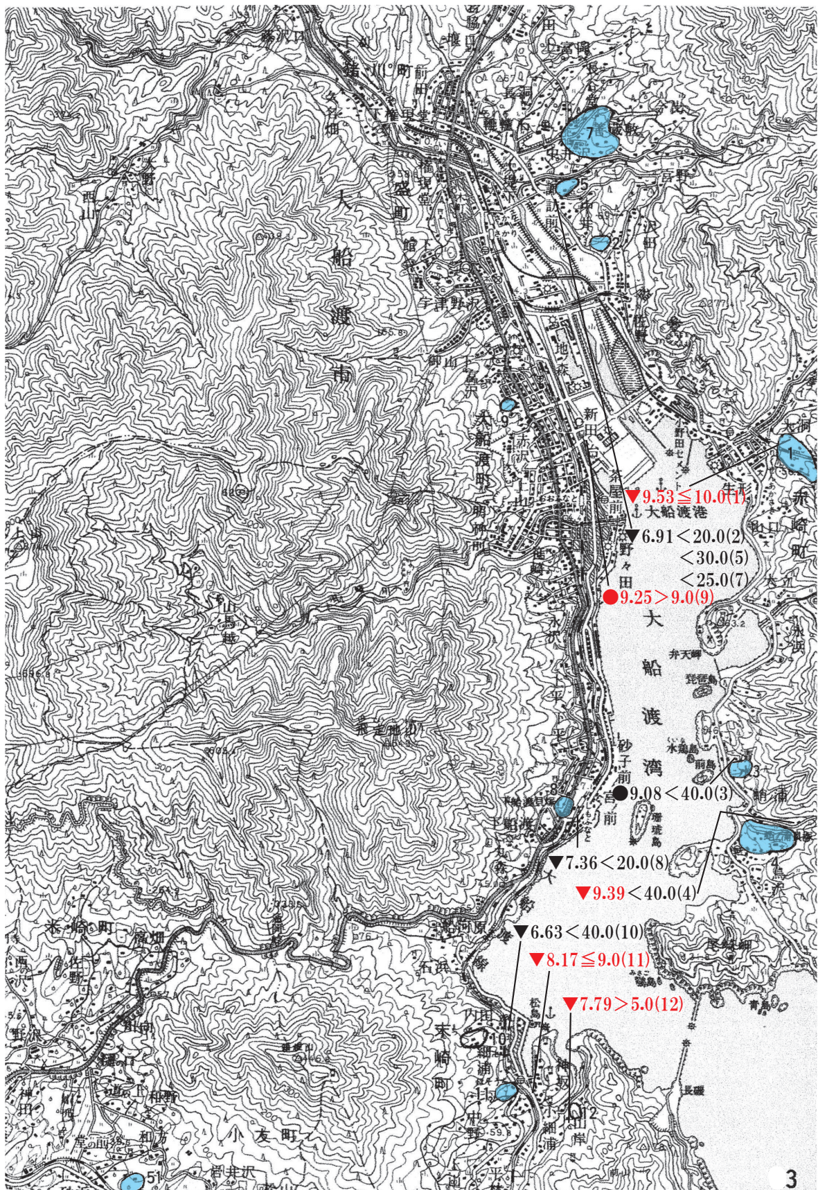
図3. 大船渡湾における縄文時代の貝塚遺跡の立地地点と東日本大震災の津波高 (《岩手県教育委員会事務局文化課 (1998) に加筆》)
