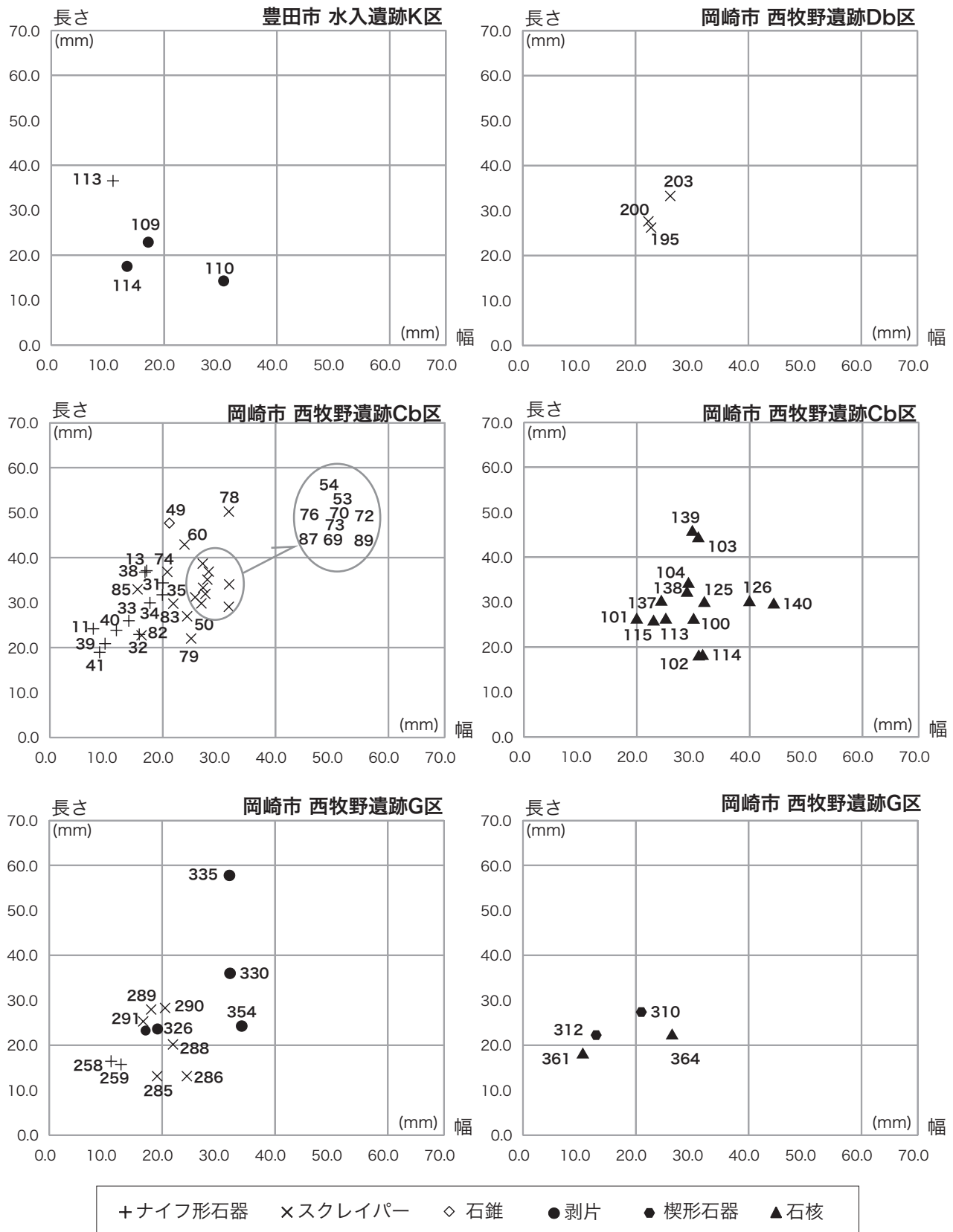
図 12 豊田市水入遺跡および岡崎市西牧野遺跡出土石器（黒曜石）法量散布図（図化報告資料分のみ） 【永井編 2005・酒井編 2013・成瀬編 2013 より、番号は各報告資料番号を示す。】
