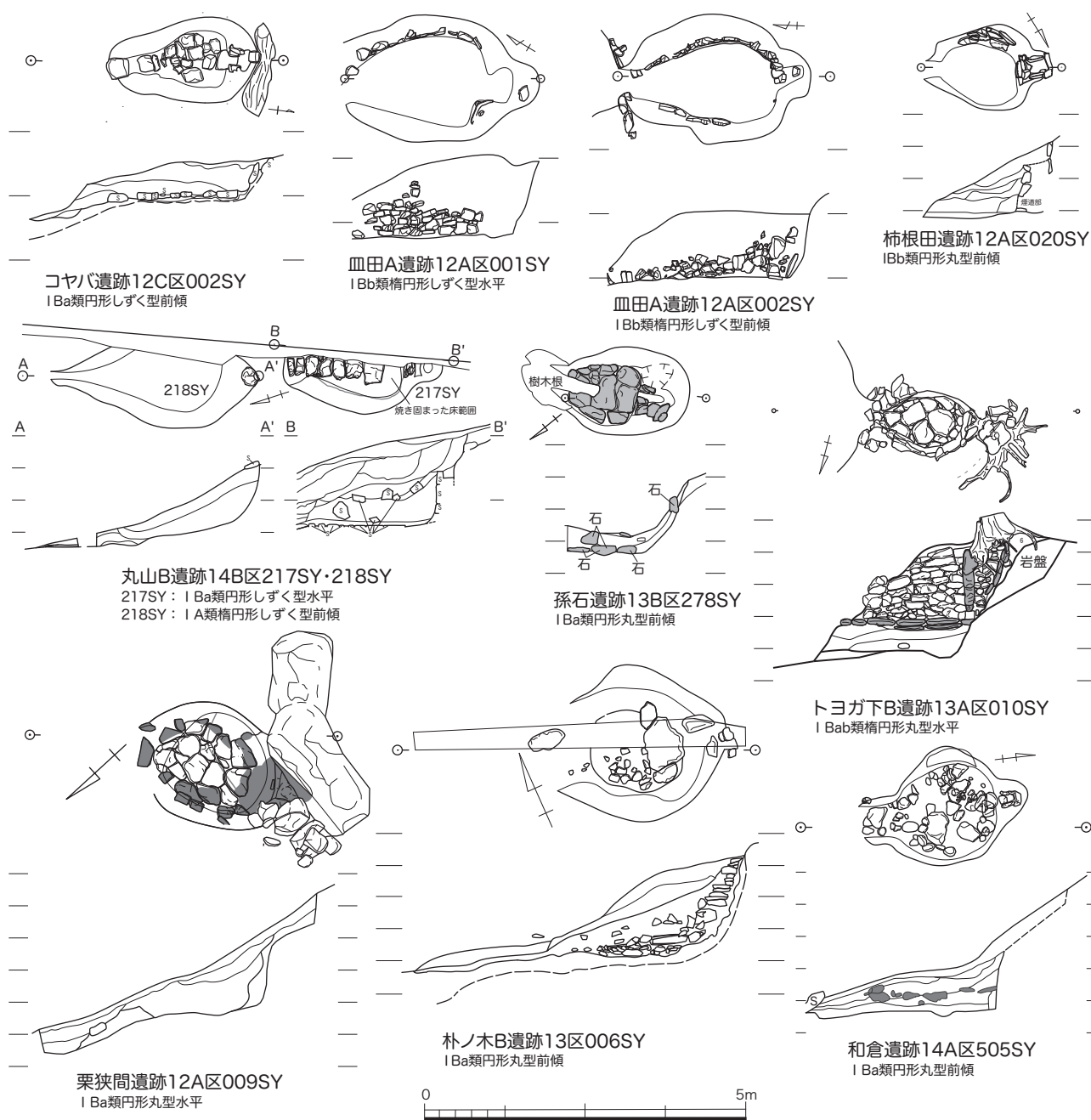
図3 炭焼窯跡 I B 類 (1:100) 【『報告書』より転載・修正】
