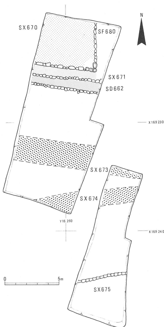
第33図 石敷広場（E・F地点）調査遺構配置図（1：200）
