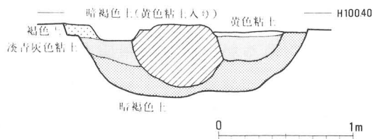
第26図 斜行溝SD755断面図(1:40)
