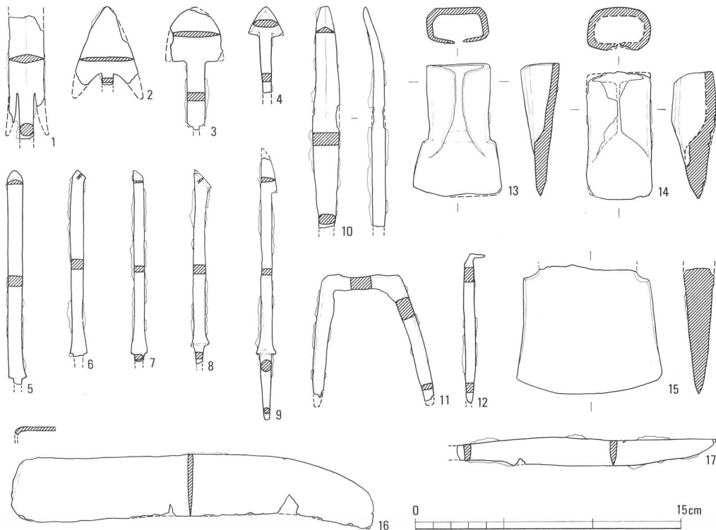
第30図 出土鉄製品（1～9；鏃，10；ヤリガンナ，11；カスガイ，12；釘，13～15；斧，16；鏃，17；刀子，1：3）
