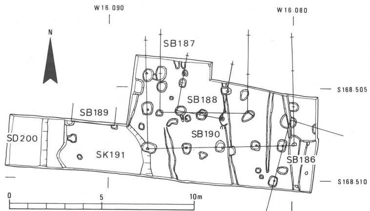
第35図 北区調査遺構配置図(1:200)
