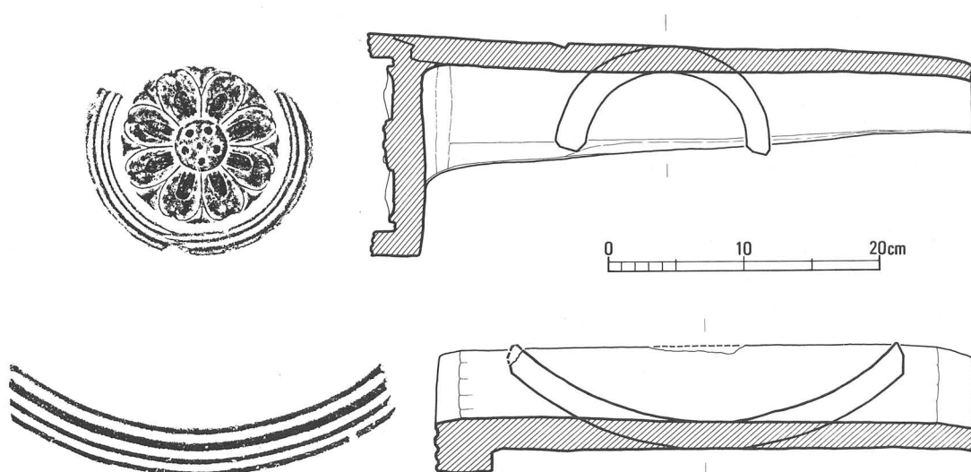
第19図 回廊所用軒瓦実測図（1：5）
