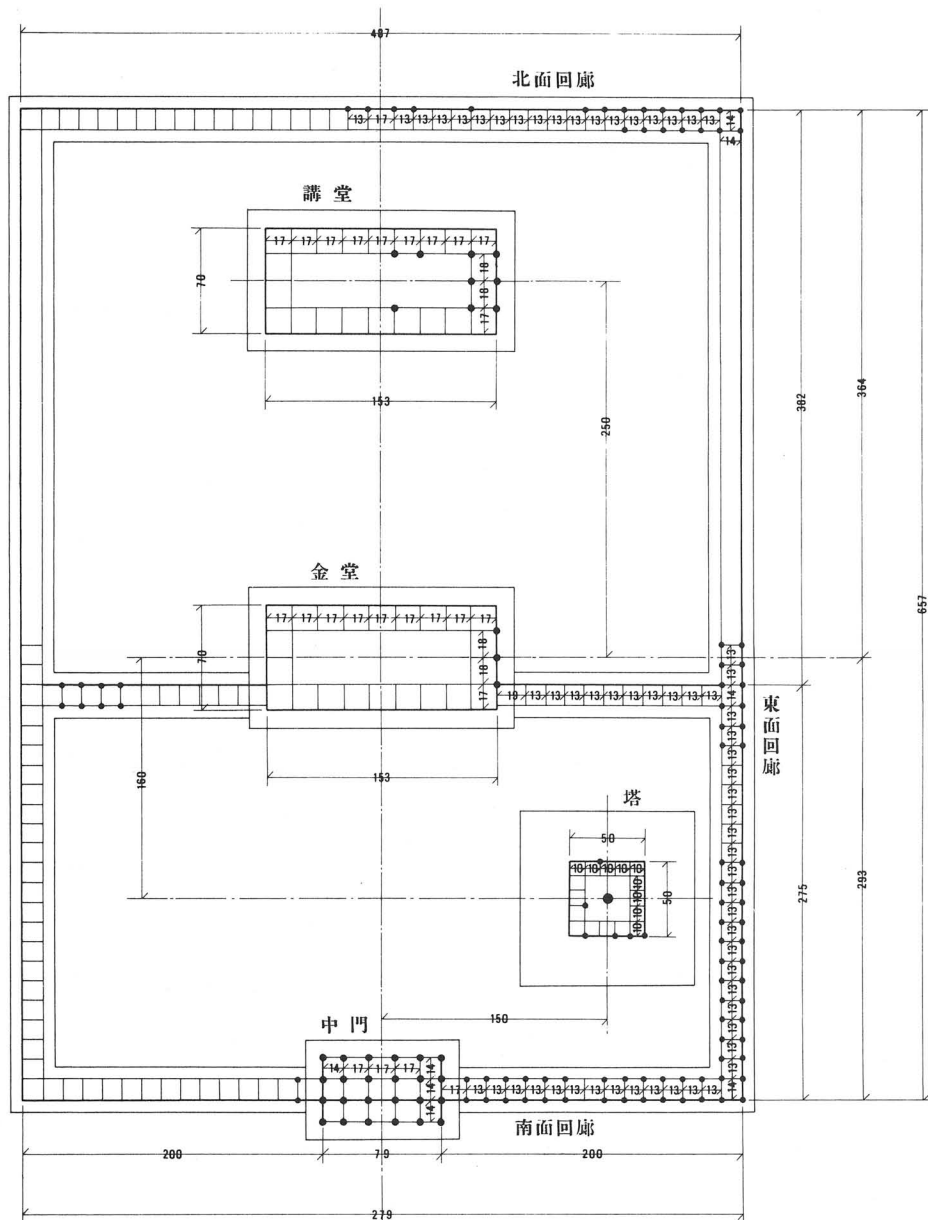
大官大寺伽藍復原図（１：１５００） 単位は大正令小尺
