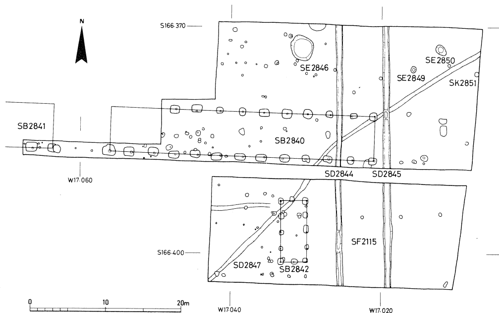
第30次調査遺構配置図（1：500）
