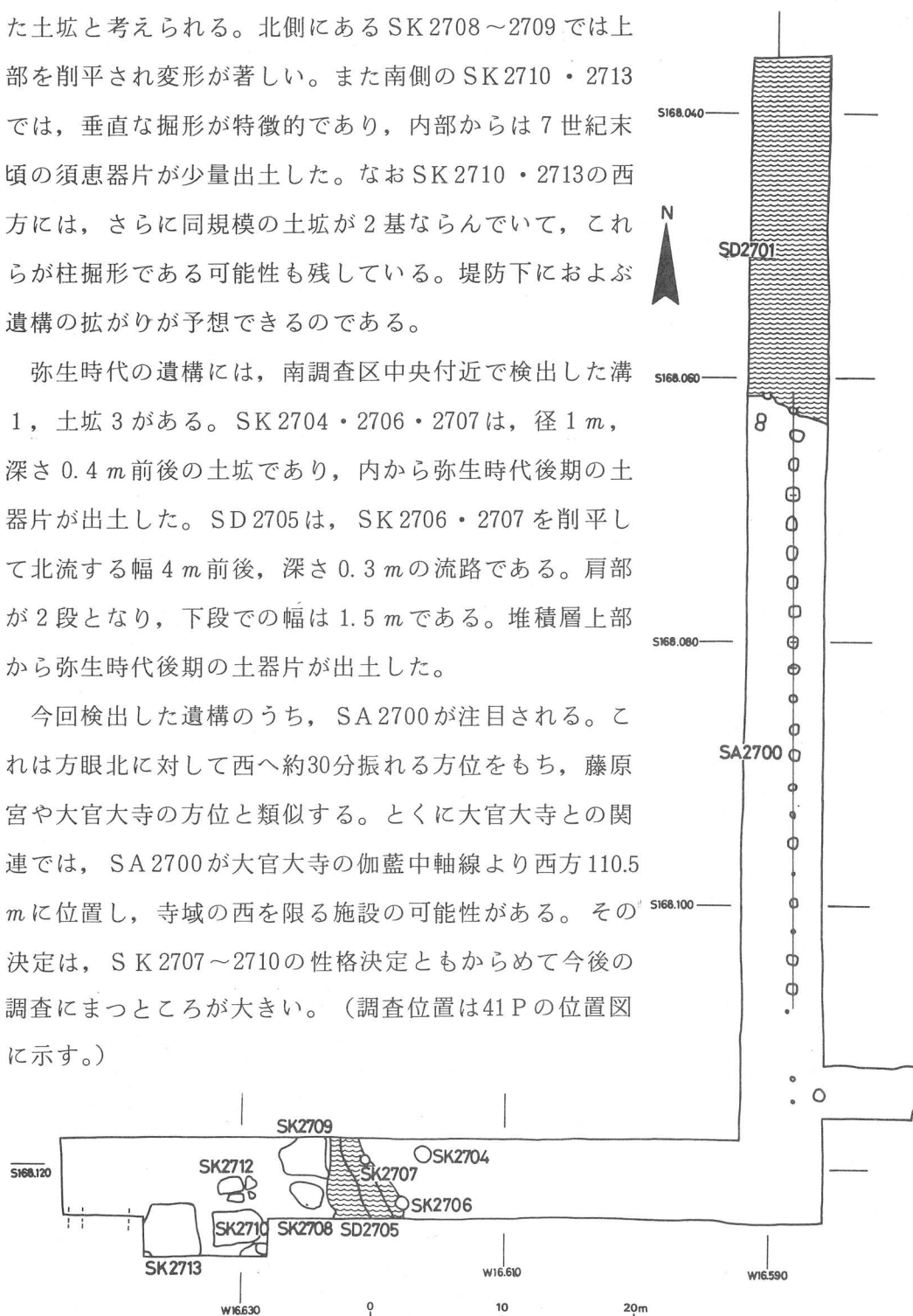
小山池調査遺構配置図（1：500）
