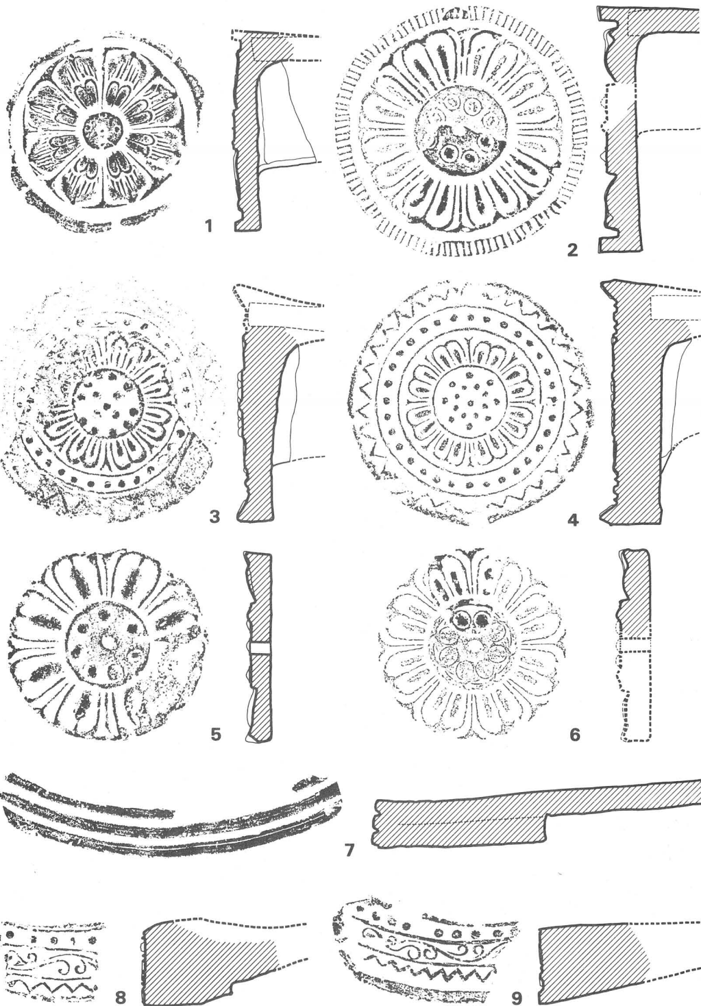
桧隈寺出土軒瓦実測図（1：4）
