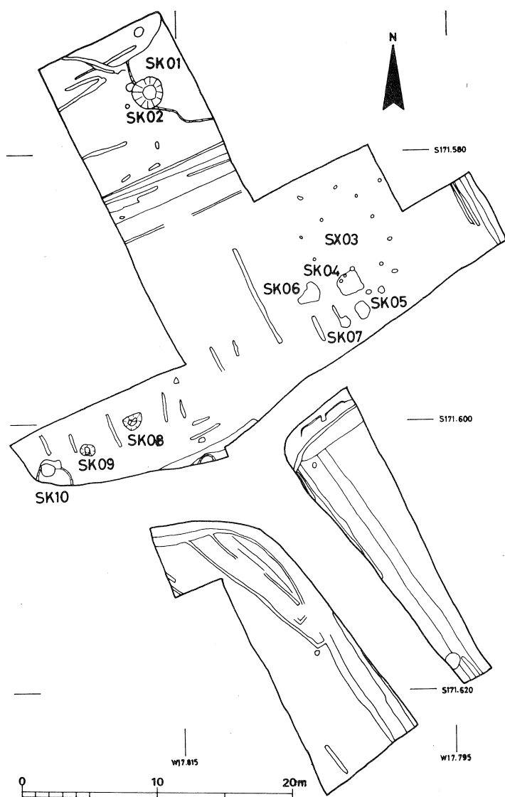
桧隈寺 第1次調査 遺構配置図 (1:400)
