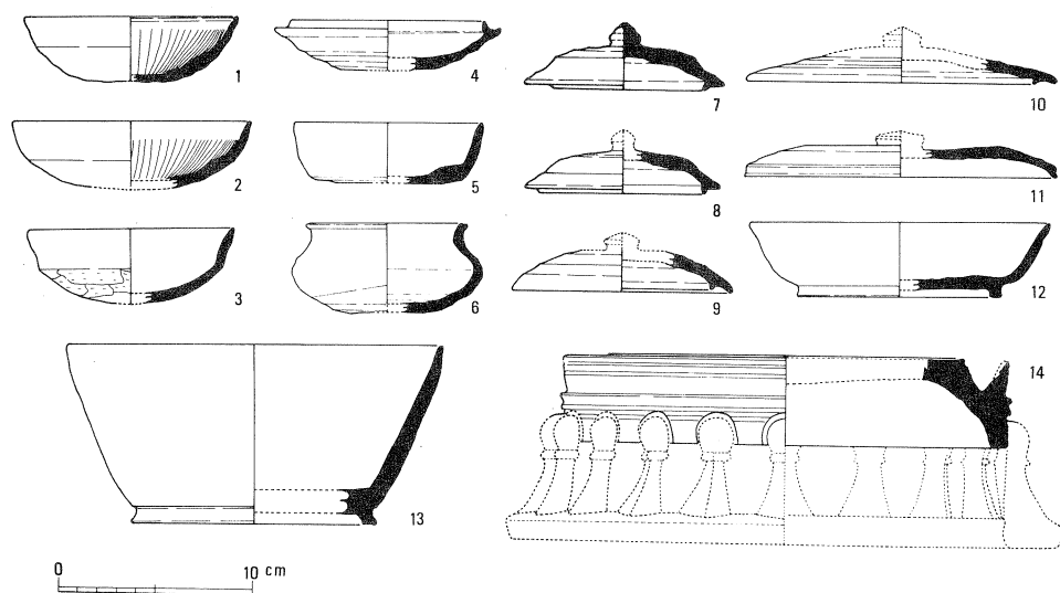
稲淵川西遺跡出土遺物実測図
