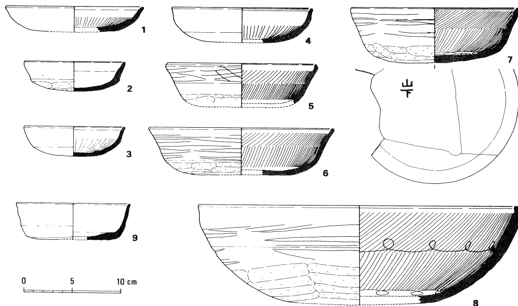
第17-2・3次調査出土土器実測図 1・3～9; S D 1951, 2; S D 1952
