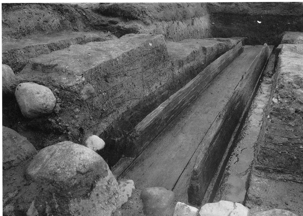
写真2 第245-2次 東面大垣の調査（木樋暗渠）
